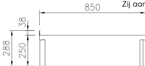
Zij aanzicht
